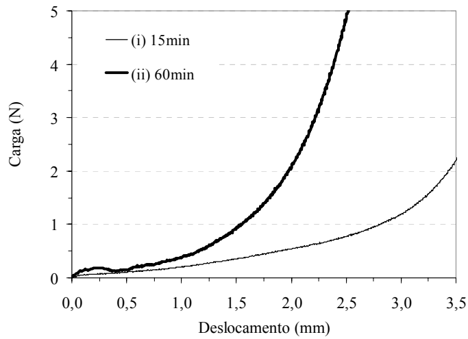
Figura 9 - Carga versus deslocamento - resultados do ensaio de squeeze-flow na pasta de cimento aos 15 min e 60 min de hidratação
