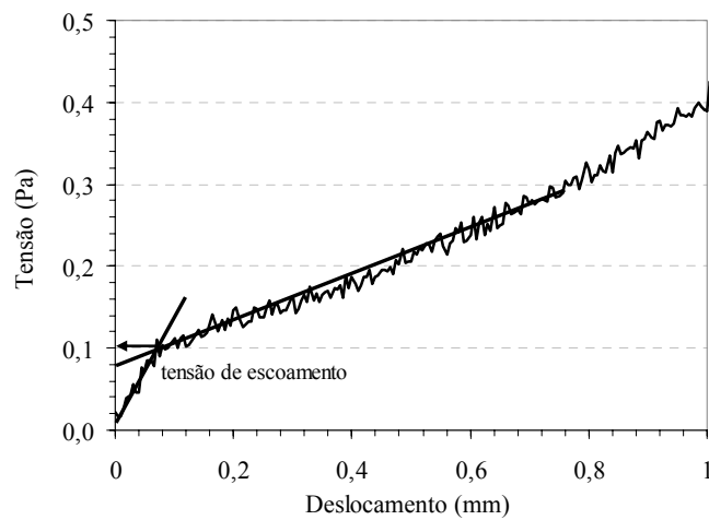
Figura 11 - Procedimento geométrico adotado para determinar a tensão de escoamento no ensaio de squeeze-flow
