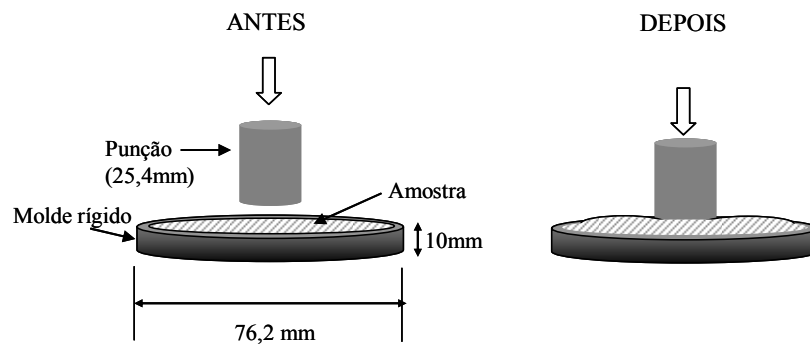
Figura 6 - Ilustração esquemática do ensaio de squeeze-flow
