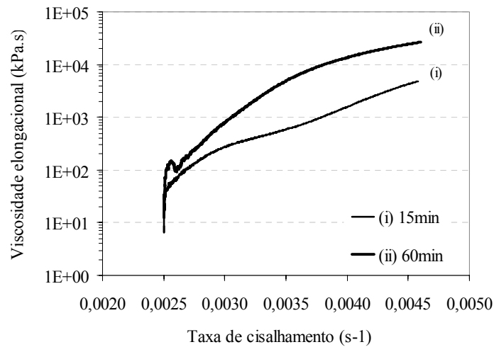
Figura 10 - Viscosidade elongacional versus taxa de cisalhamento elongacional para a pasta de cimento aos 15 min e 60 min de hidratação
